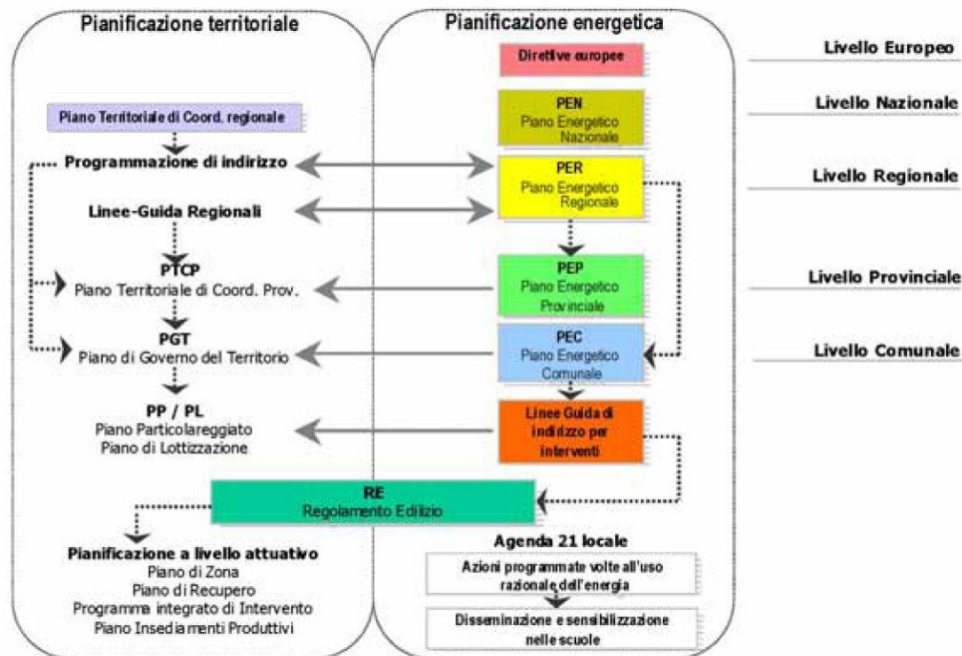
Figura 56: Schema pianificazione energetica
