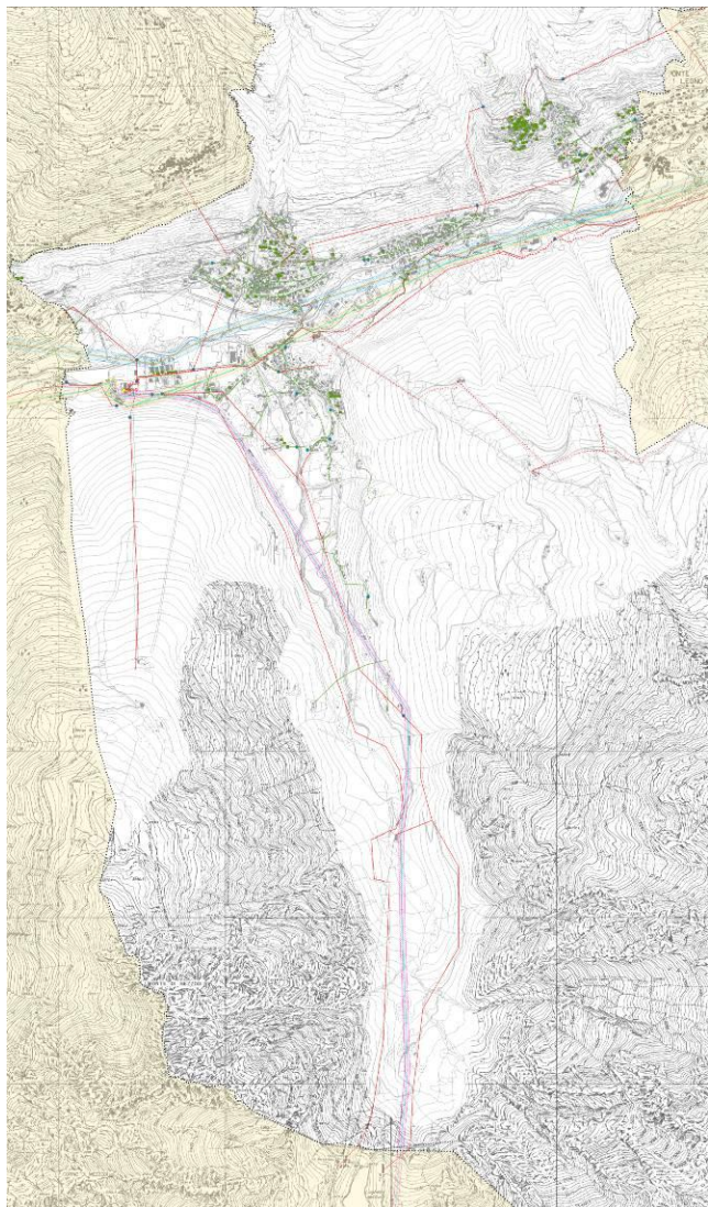
Figura 57: Estratto della tavola degli elettrodotti a Temù.
