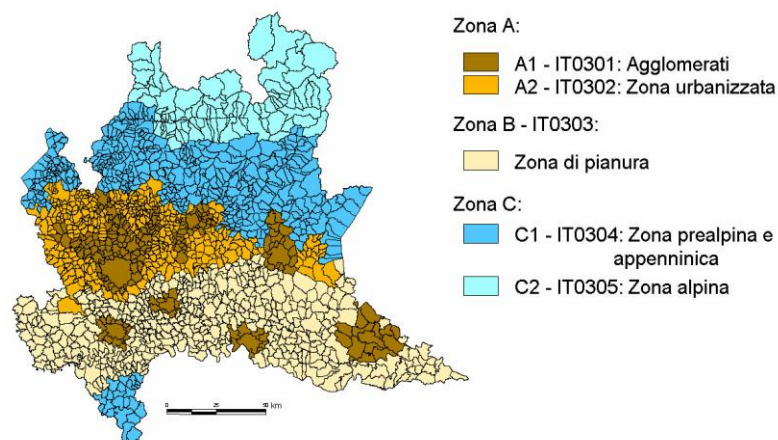
Figura 12: Zonizzazione regionale per la qualità dell'aria
