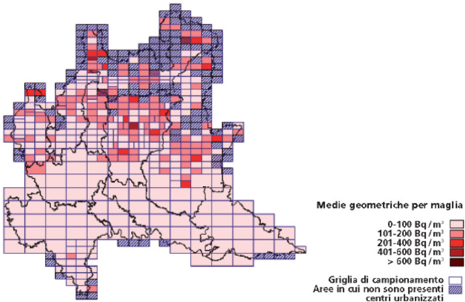
Figura 62: Aree territoriali a maggior presenza di radon (Fonte Arpa)
