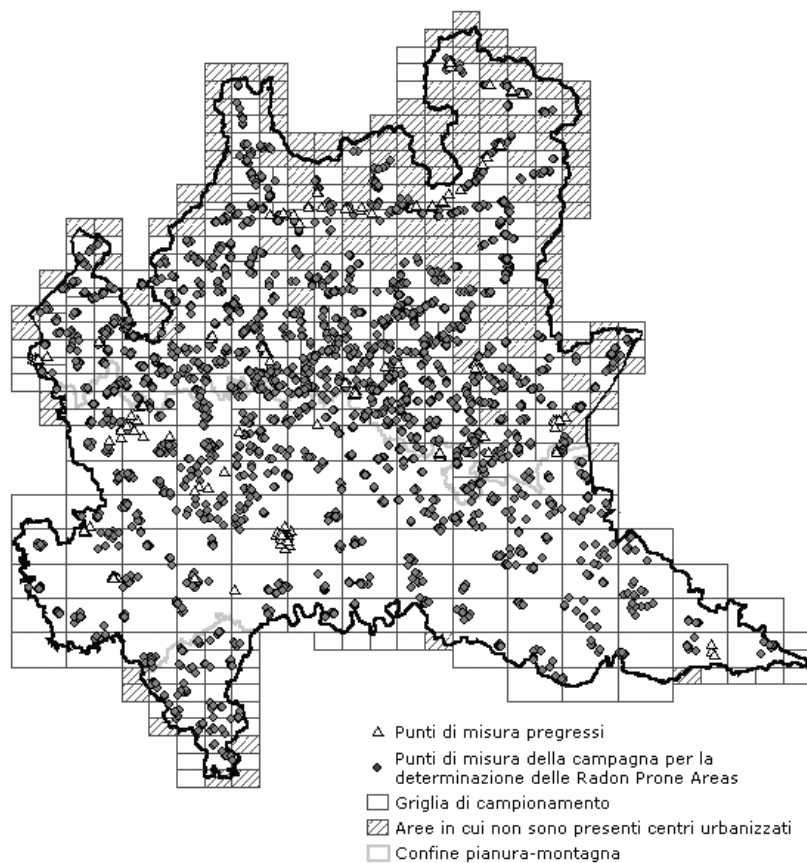
Figura 61: Piano di mappatura per la determinazione delle radon prone areas in Lombardia (2003-2005) – localizzazione dei punti di misura. Sono stati individuati da 5 a 10 punti di misura in ogni maglia nella quale siano presenti centri urbanizzati.
