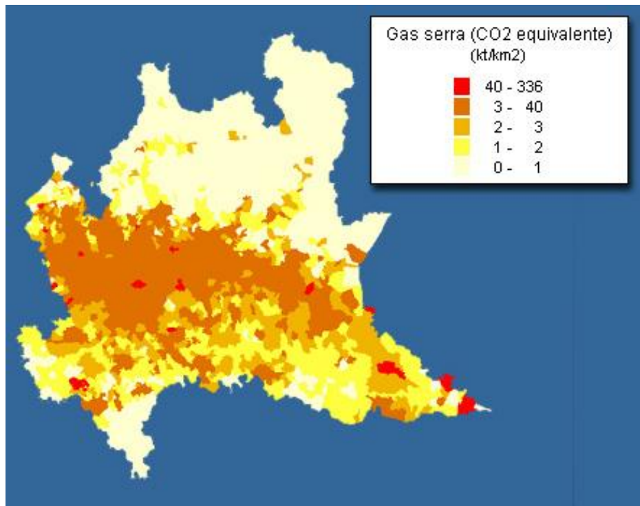
Figura 16: Emissioni di inquinanti in Regione Lombardia
