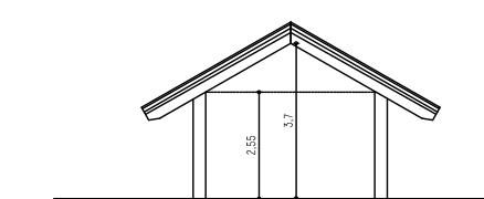
SEZIONE TRASVERSALE
